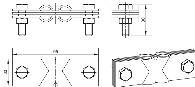
Рисунок / Figure 1 – Габаритные размеры / Overall dimensions
